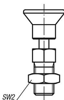
Forma B senza incavo d'arresto con controdato
