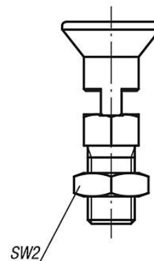
Forma D con incavo d'arresto con controdato
