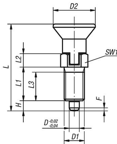
Forma C con incavo d'arresto senza controdato
