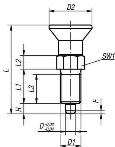
Forma A senza incavo d'arresto senza controdato
