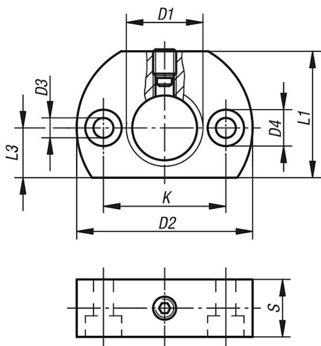
Forma A foro di montaggio parallelo alla spina a leva
