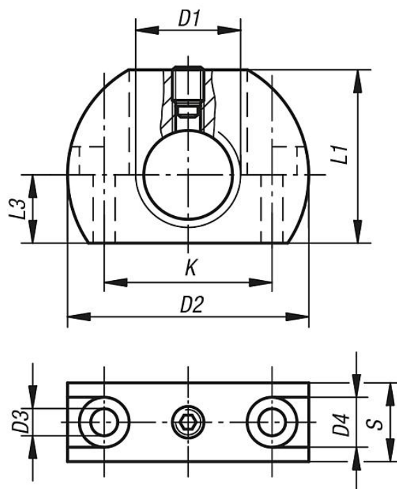
Forma B foro di montaggio perpendicolare alla spina a leva
